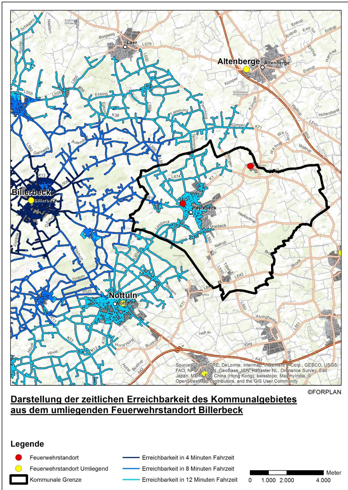
Abb. 6.9 Fahrzeitsimulation Billerbeck
