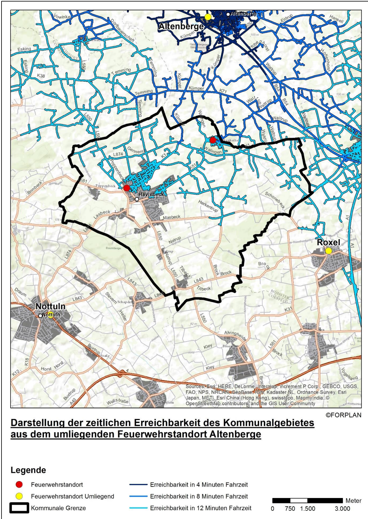
Abb. 6.8 Fahrzeitsimulation Altenberge
