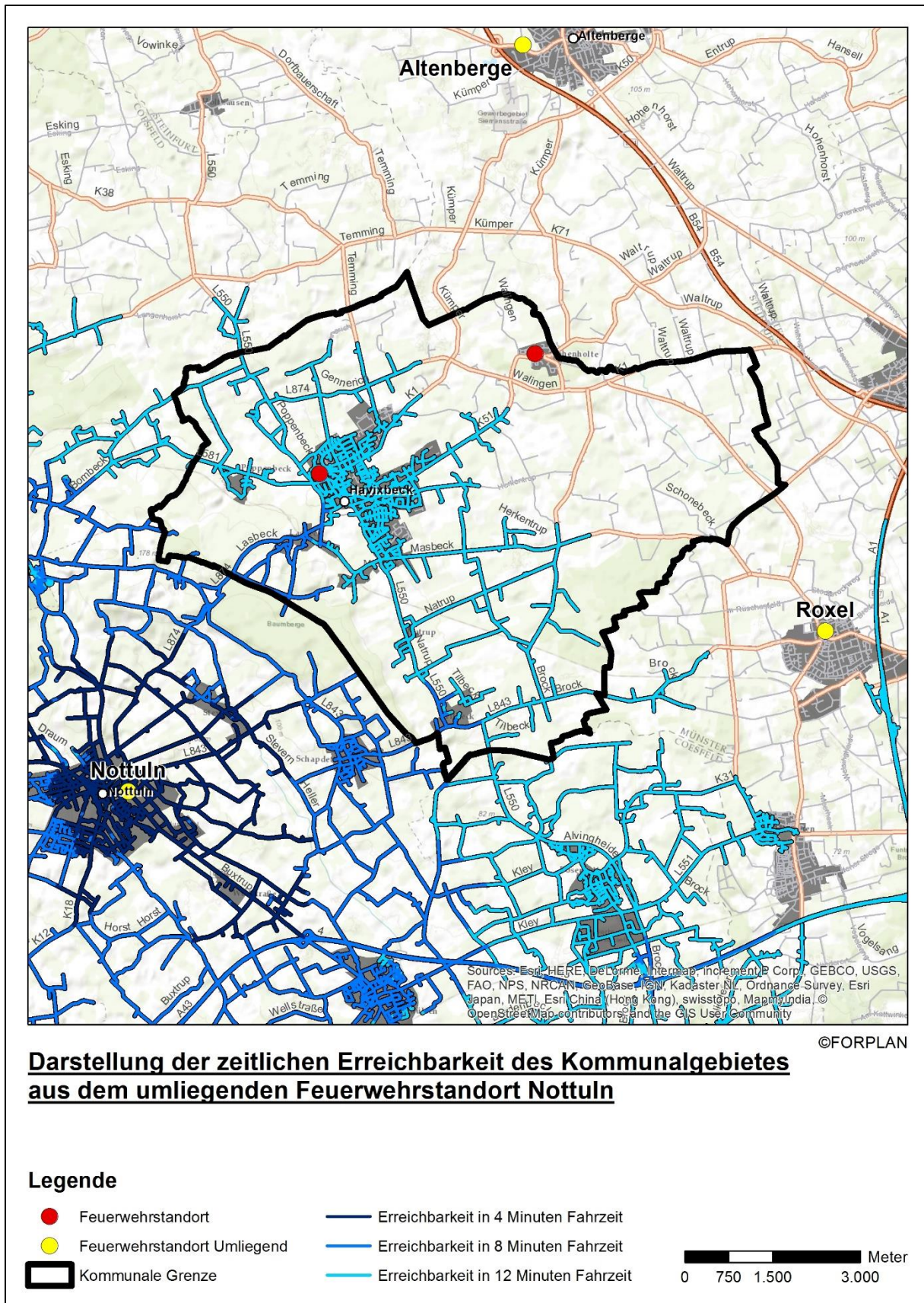
Abb. 6.10 Fahrzeitsimulation Nottuln
