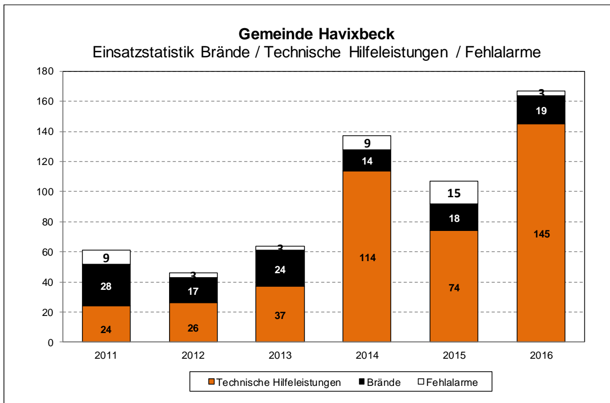
Abb. 6.1 Einsatzstatistik
