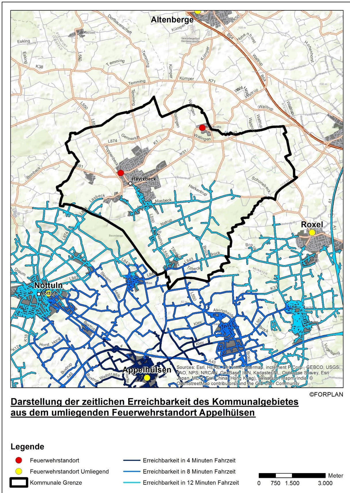
Abb. 6.11 Fahrzeitsimulation Appelhülsen
