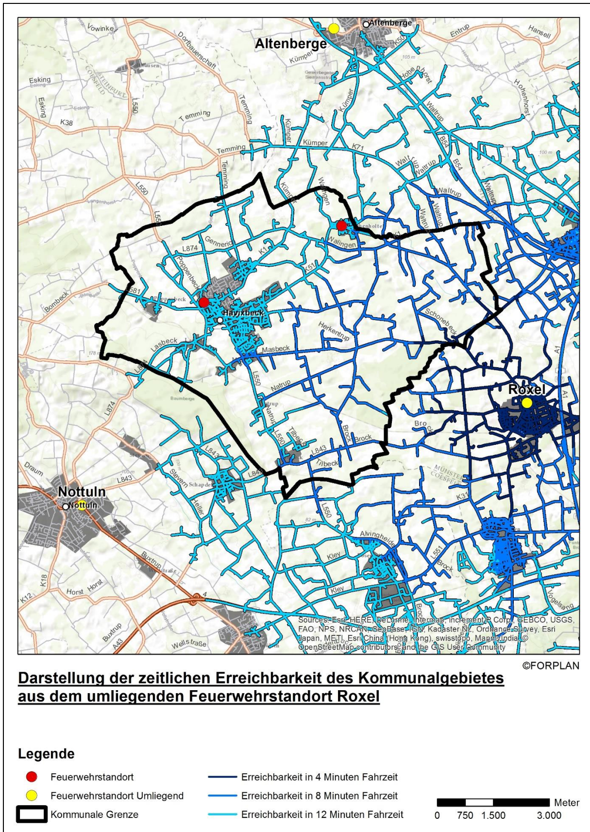
Abb. 6.12 Fahrzeitsimulation Roxel
